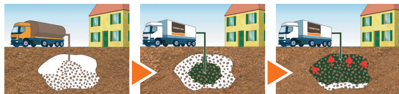
Comblement avec des billes d'argile expansée
